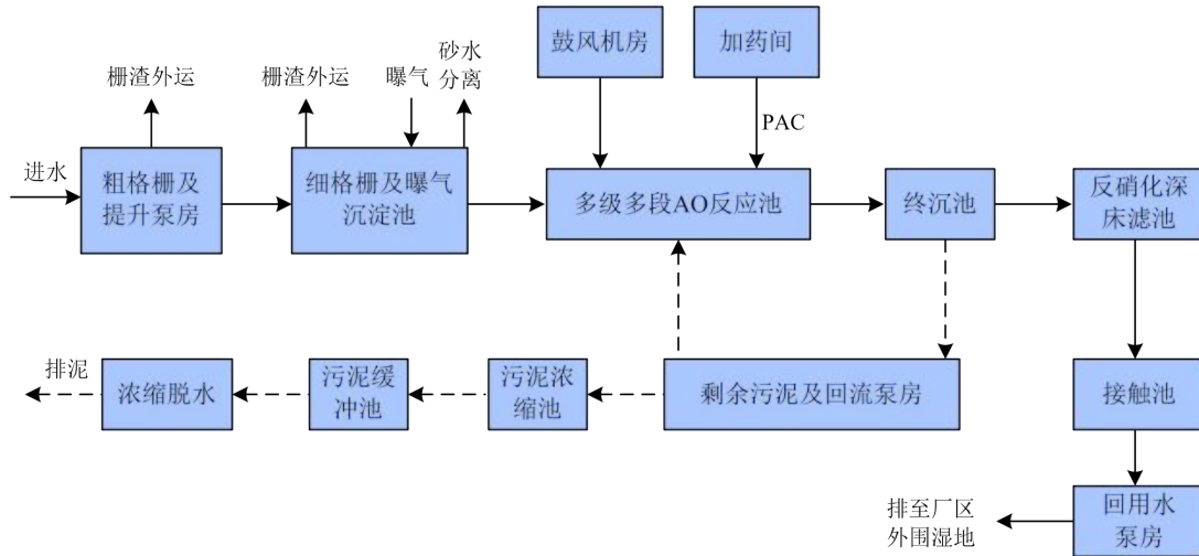
图 2.2-2 二期工程污水处理工艺流程图
