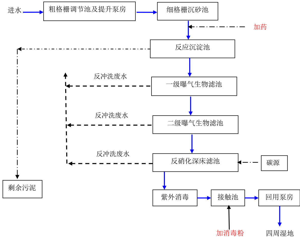
图 2.2-1 一期工程污水处理工艺流程图
